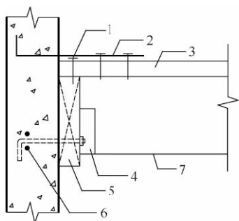
图 7.3.7 木楼盖作为墙体侧向支撑示意
