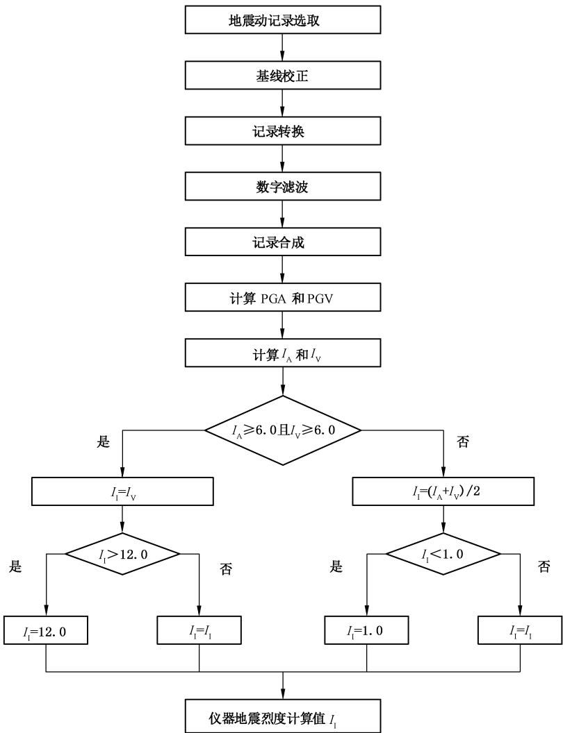
图 A.1 地震烈度的仪器测定流程图
